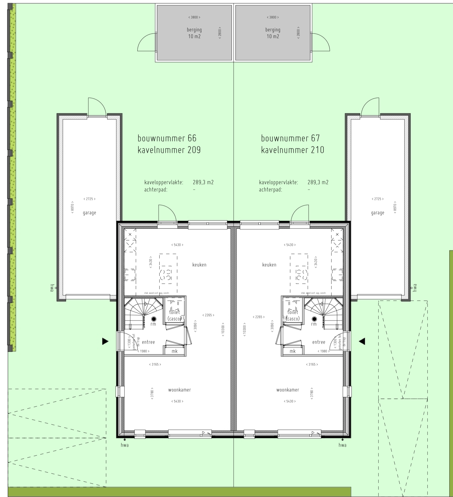
BEGANE GROND 2kap - 209 t/m 210
