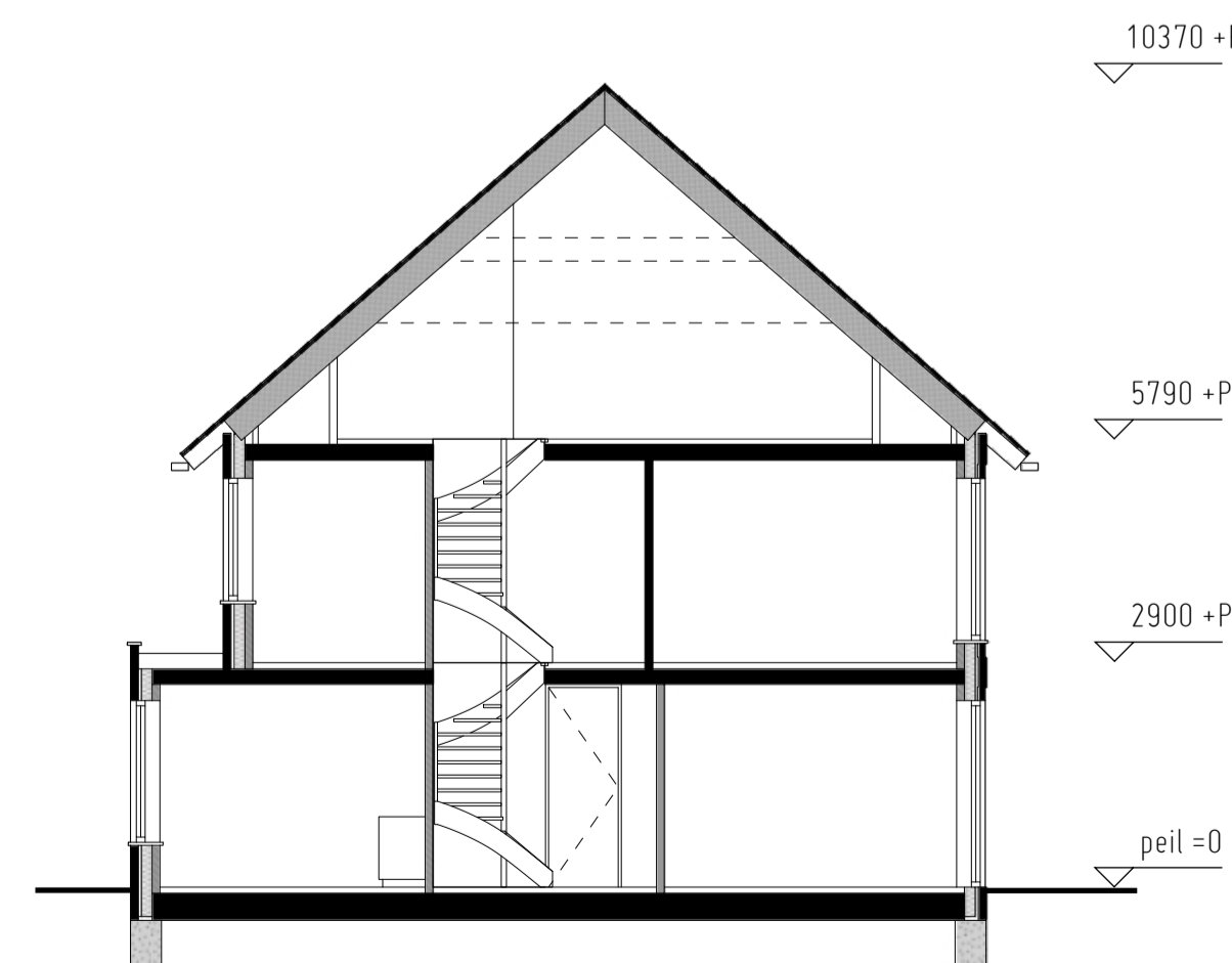
DOORSNEDE
