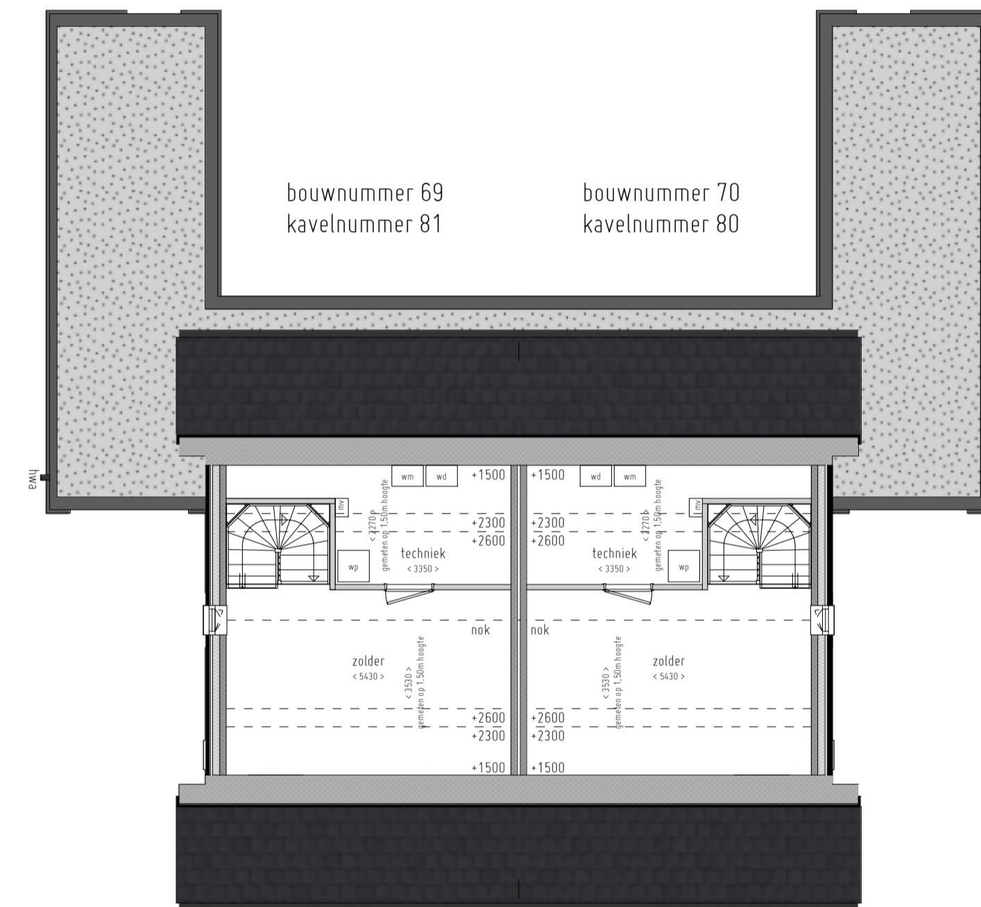
ZOLDER 80 t/m 81
