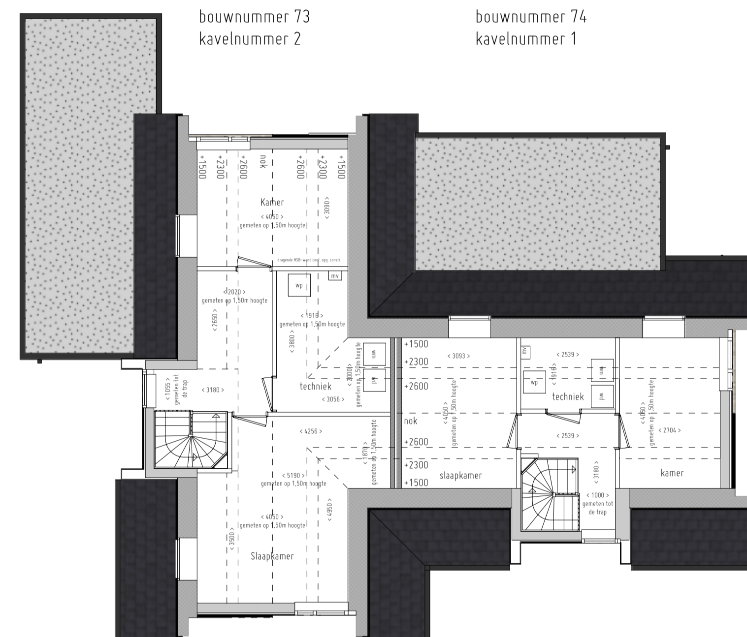
EERSTE VERDIEPING 1 t/m 2
