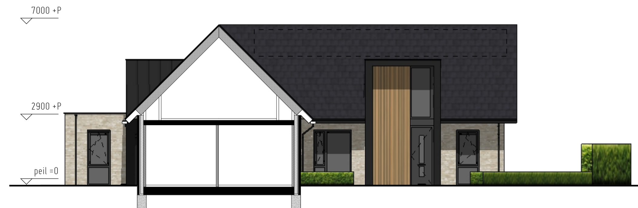
DOORSNEDE
